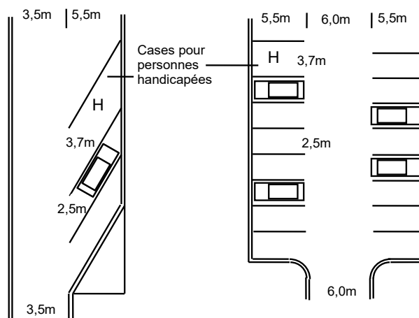
STATIONNEMENT À 60° STATIONNEMENT À 90°
